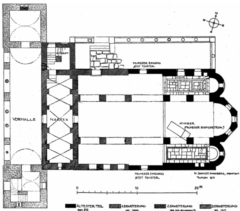
План на църквата от арх. М. Шмит-Анаберг
