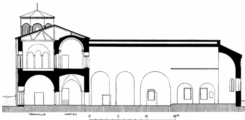
„Света София“, Охрид Нагълъжен разрез Чертеж архитект М. Шмит-Анаберг
