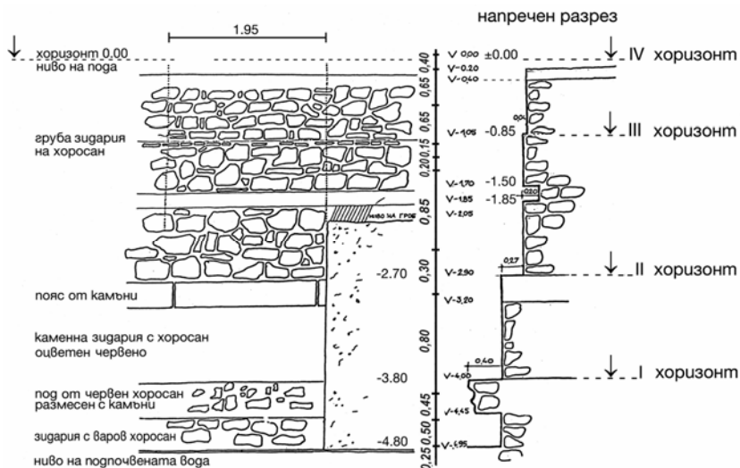
Сондаж при външната северна стена на наоса (по арх. Борис Чипан)
