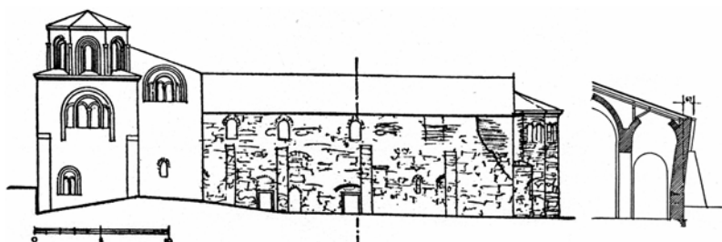
Охрид, „Света София“ Южна фасада и разрез през южния кораб Състояние на сградата в 1950 година Чертеж: ЮНЕСКО
