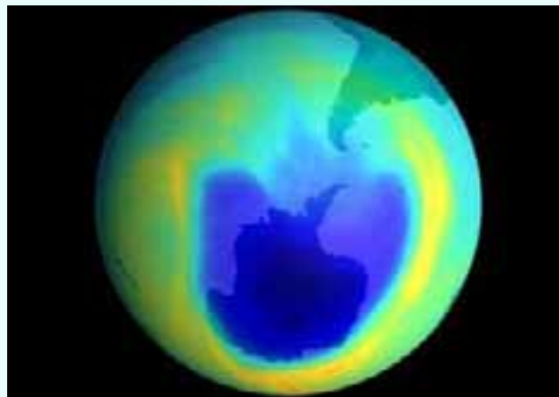
Озонска дупка над Антарктикот
