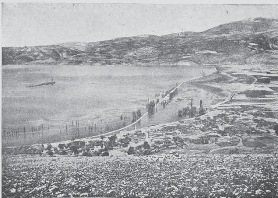
Островското езеро.
